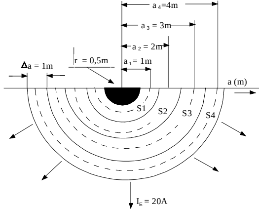
Şekil-T.1 Bir yarımküre topraklayıcıdan akımın toprağa yayılması
