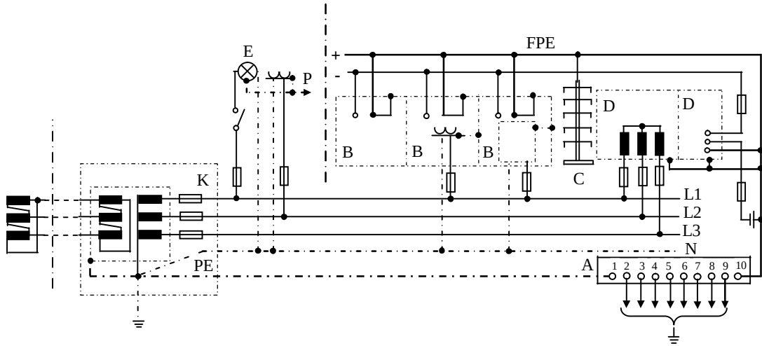
Şekil-16 Madde 21-b1'de belirtilen bir iletişim sisteminin fonksiyon ve koruma topraklamasına örnek (Not: Bu şekil mecburi olmayıp, yalnızca bir fikir vermek amacıyla taşımaktadır.)
