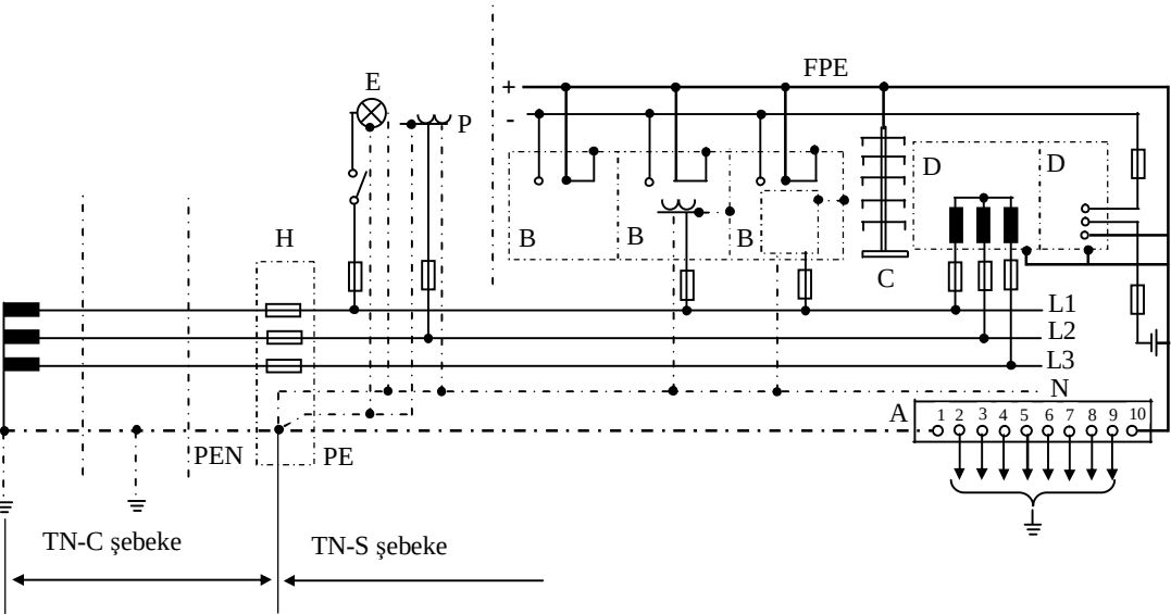
Şekil-18 Madde 21-b3'de belirtilen bir iletişim tesisinin fonksiyon ve koruma topraklamasına örnek (Not: Bu şekil mecburi olmayıp, yalnızca bir fikir vermek amacını taşımaktadır.)
