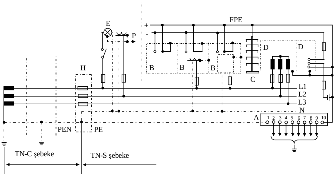
Şekil-17 Madde 21-b2'de belirtilen bir iletişim tesisinin fonksiyon ve koruma topraklamasına örnek (Not: Bu şekil mecburi olmayıp, yalnızca bir fikir vermek amacını taşımaktadır.)
