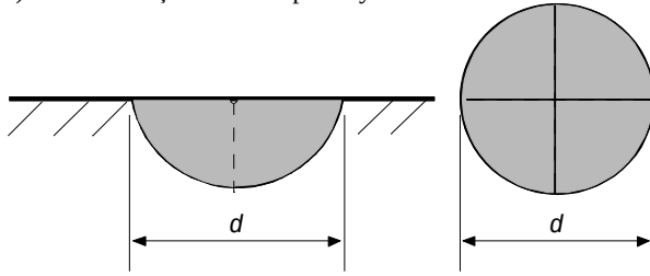
Şekil-T.14 Yarım küre şeklindeki topraklayıcı
