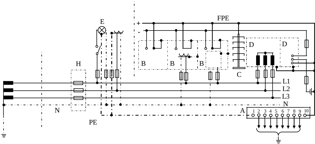
Şekil-20 Madde 21-c2'de belirtilen bir iletişim tesisinin fonksiyon ve koruma topraklamasına örnek (Not: Bu şekil mecburi olmayıp, yalnızca bir fikir vermek amacıyla taşınmaktadır.)
