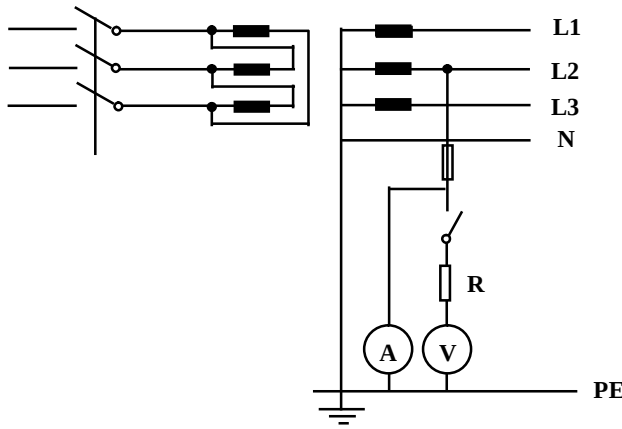
Şekil-N.2 Arıza çevrim (halka) empedansının gerilim düşümü yardımı ile ölçülmesi deneyi
