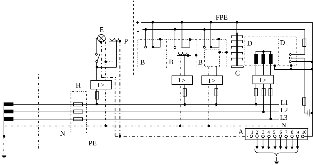
Şekil-19 Madde 21-c1'de belirtilen bir iletişim tesisinin fonksiyon ve koruma topraklamasına örnek (Not: Bu şekil mecburi olmayıp, yalnızca bir fikir vermek amacıyla taşınmaktadır.)
