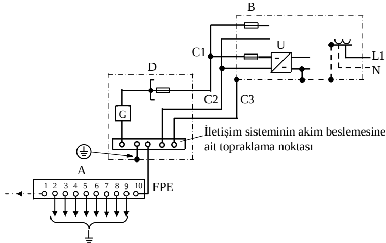
Şekil-15 İletişim sistemine ilişkin akım beslemesinin anma gerilimleri sınırlanmaksızın bir iletişim tesisi için ek topraklama iletkeni ile yapılan işletme ve koruma topraklamasına örnek (Not: Bu şekil mecburi olmayıp, yalnızca bir fikir vermek amacıyla taşımaktadır.)
